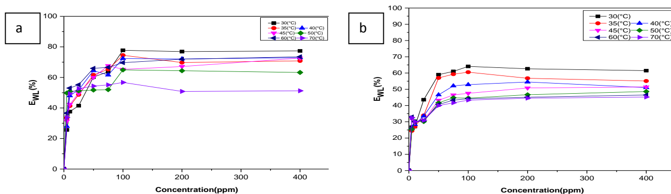
Figure IV.7 : Efficacité d'inhibition en fonction de la concentration de l'acier DC06EK dans la solution H 2 SO 4 (0,1 M), en présence du tryptophane (a) et la proline (b) à différentes températures.
