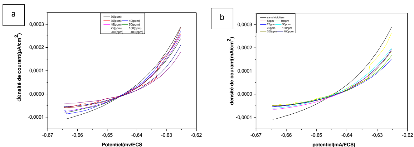
Figure IV.20. Les Courbes de polarisation de R_p (a :tryptophane+NaI, b :Proline +NaI), obtenues à \pm 20 mV/ECS de l'acier DC06EK immergé dans H_2SO_4 (0.1 M).
