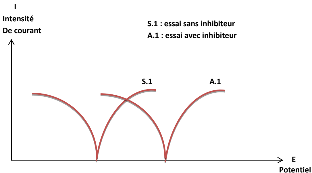
Figure I.5. Effet de l'inhibiteur anodique sur la courbe de polarisation de l'acier [7] .
