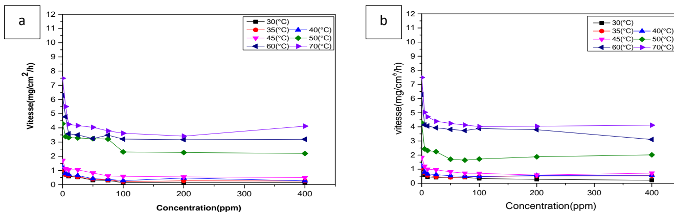
Figure IV.14. Vitesse d'inhibition en fonction de la concentration de l'acier DC06EK dans la solution H_2SO_4 (0,1 M), en présence de ( a :Tryptophane+5ppm NaI, b :Proline+5ppm NaI), à différentes températures
