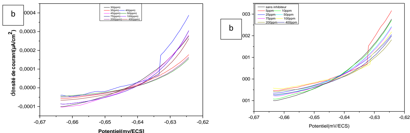
Figure IV.12. Les Courbes de polarisation de Rp (a :tryptophane, b :Prolinene), obtenues à ± 20 mV/ECS de l’acier DC06EK immergé dans H 2 SO 4 (0.1 M).
