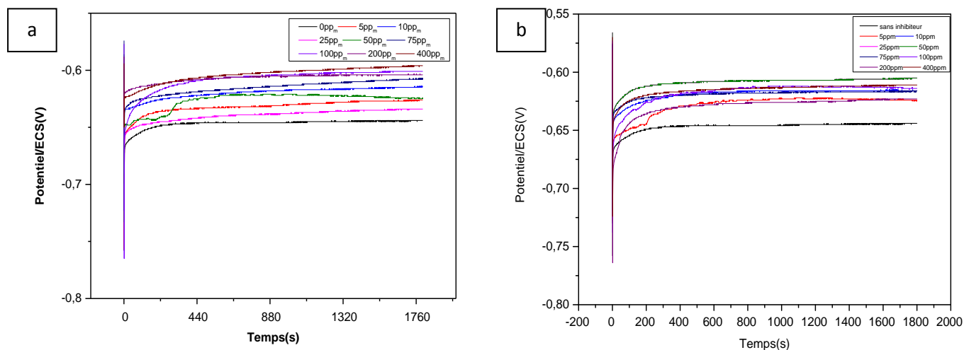
Figure IV.10. Chronopotentiogrammes de l'acier DC06EK dans une solution de H_2SO_4 (0,1M), de différentes concentrations en produits inhibiteurs (a :tryptophane, b :proline).
