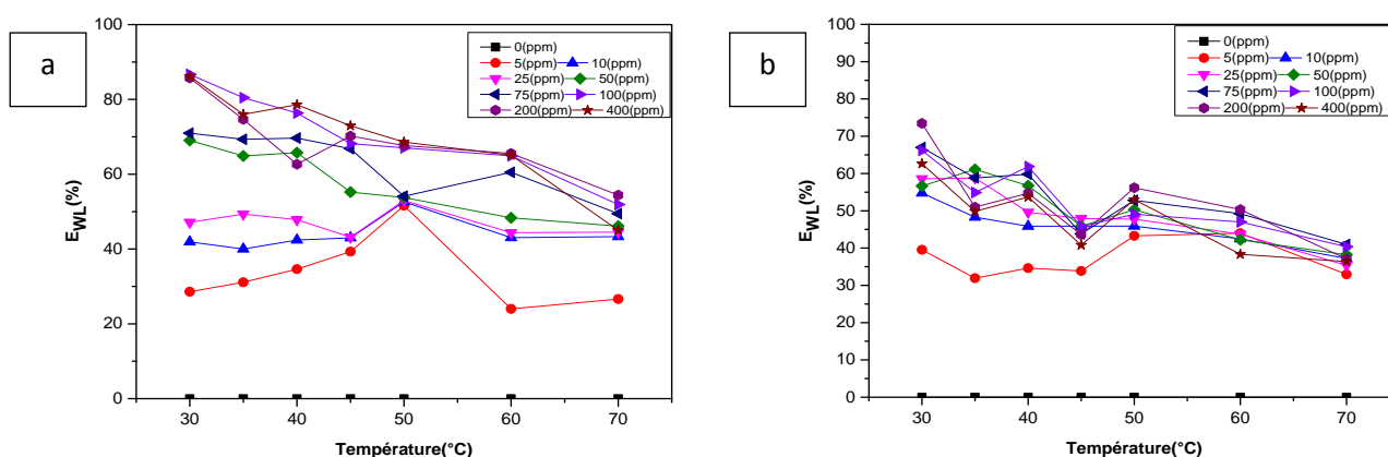
Figure IV.17. Efficacité d'inhibition en fonction de la température de l'acier DC06EK dans la solution H_2SO_4 (0,1 M), en présence de (a : Tryptophane+5ppm NaI, b : Proline+5ppm NaI), à différentes concentrations
