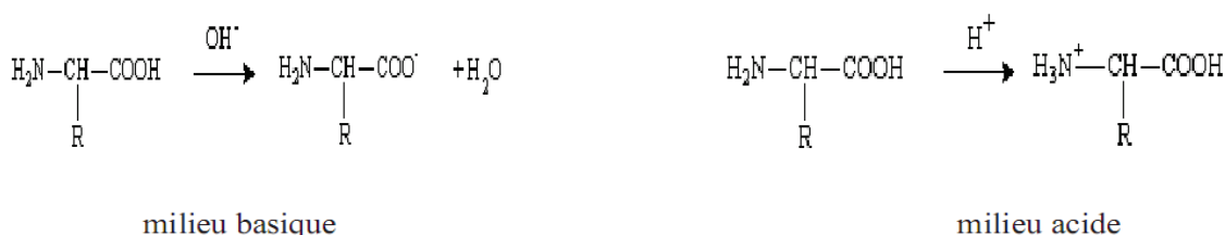
Figure II.2. Les propriétés acido-basiques des acides aminés. [62]
