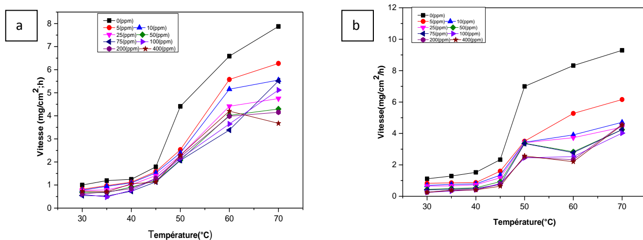
Figure IV.6. Vitesse d'inhibition en fonction de la température de l'acier DC06EK dans la solution H_2SO_4 (0,1 M), en présence de (b : Proline , a : Tryptophane ) à différentes concentrations.
