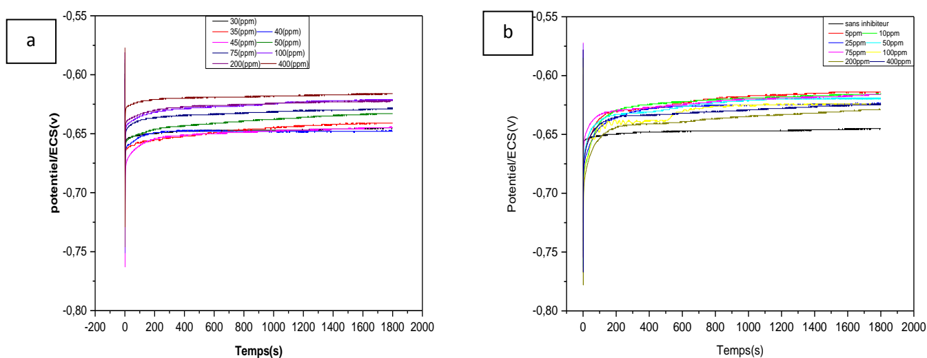
Figure IV.18. Chronopotentiogrammes de l'acier DC06EK dans une solution de H_2SO_4 (0,1M), Contenant différentes concentrations en produits inhibiteurs (a : Tryptophane +NaI et b : Proline+NaI ).
