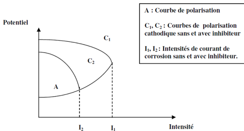
Figure I.6. Effet de l'inhibiteur cathodique sur la courbe de polarisation de l'acier [23] .
