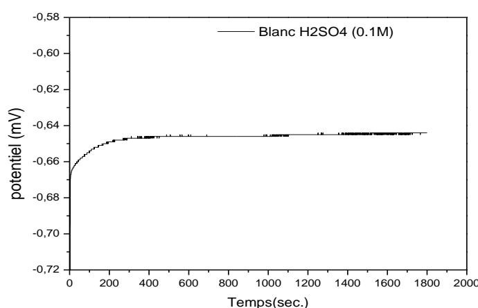
Figure IV.9. Chronopotentiogramme de l'acier DC06EK dans une solution Aérée de H_2SO_4 (0.1M) Sans inhibiteur.
