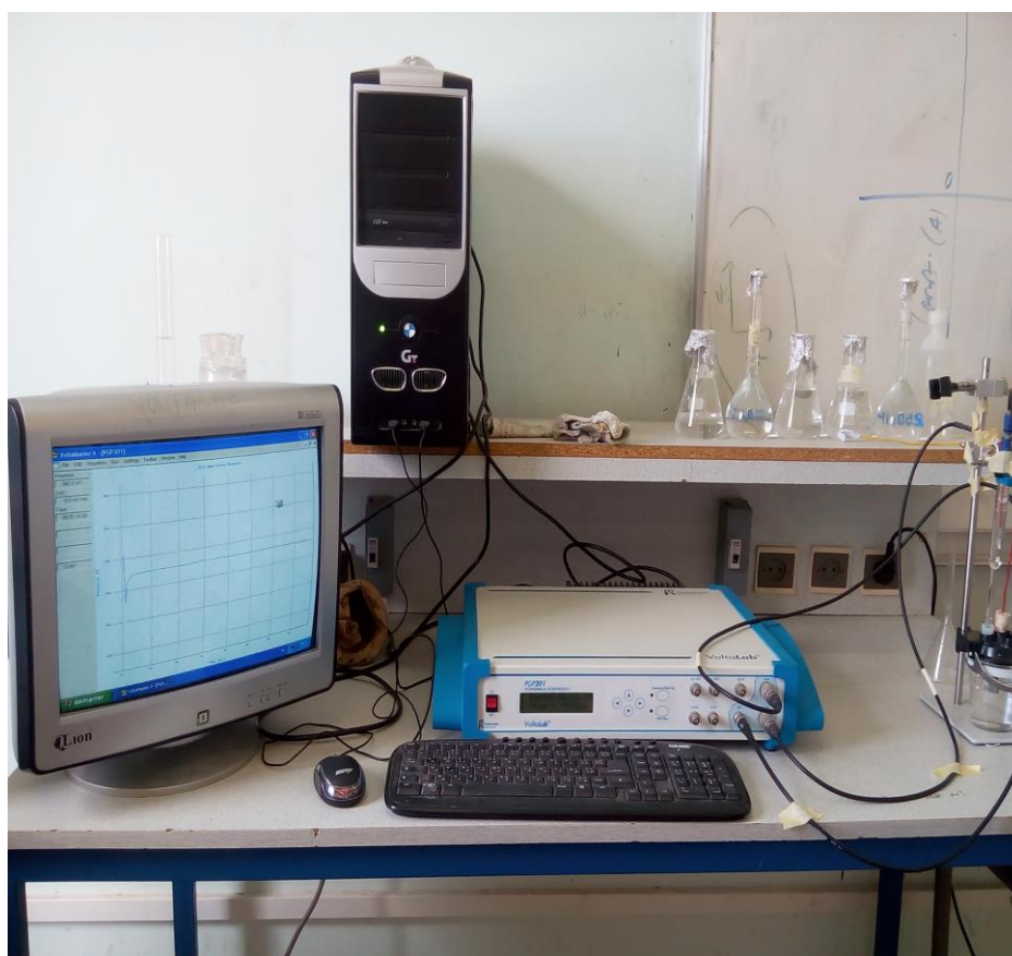
Figure III.4. Image photographique du potentiostat/Galvanostat voltalab21, utilisé.
