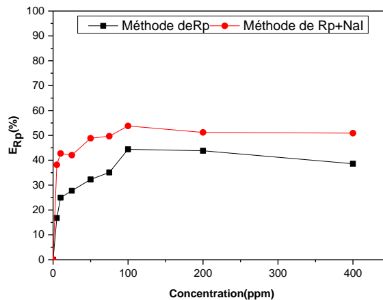
Figure IV.22 : Efficacité d'inhibition, évalué par les trois méthodes de ( a : gravimétrie , b : tafel, et c : Rp) en fonction de la concentration de ( Proline et Proline +5ppm Na I ).
