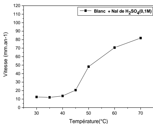
Figure IV.13. Vitesse de corrosion en fonction de la température de l'acier DC06EK dans la solution H_2SO_4 (0,1 M) + 5 ppm (NaI).
