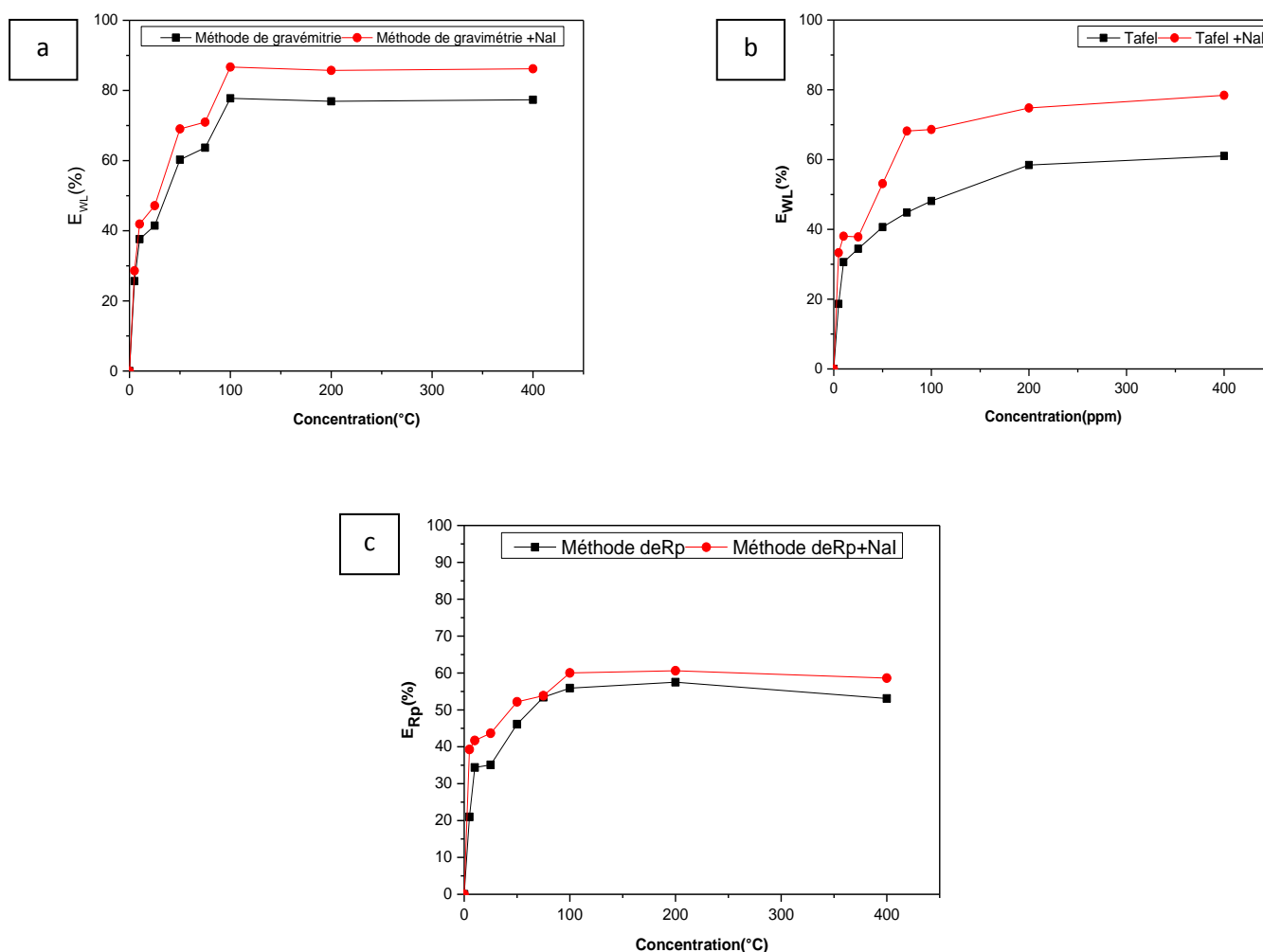
Figure IV.21 : Efficacité d'inhibition, évalué par les trois méthodes de ( a : gravimétrie , b : tafel , c : Rp ) en fonction de la concentration de (Tryptophane et Tryptophane +5ppm Na I).
