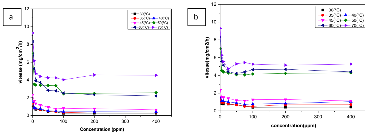
Figure IV.5. Vitesse d'inhibition en fonction de la concentration de l'acier DC06EK dans la solution H_2SO_4 (0,1 M), en présence de (a : Tryptophane , b : Proline ) à différentes températures.
