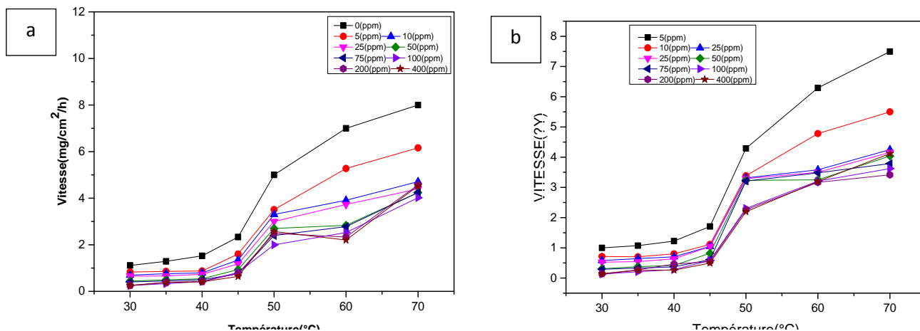
Figure IV.15. Vitesse d'inhibition en fonction de la température de l'acier DC06EK dans la solution H 2 SO 4 (0,1 M), en présence de ( a :Proline+5ppm NaI, b : Tryptophane+5ppm NaI), à différentes concentrations
