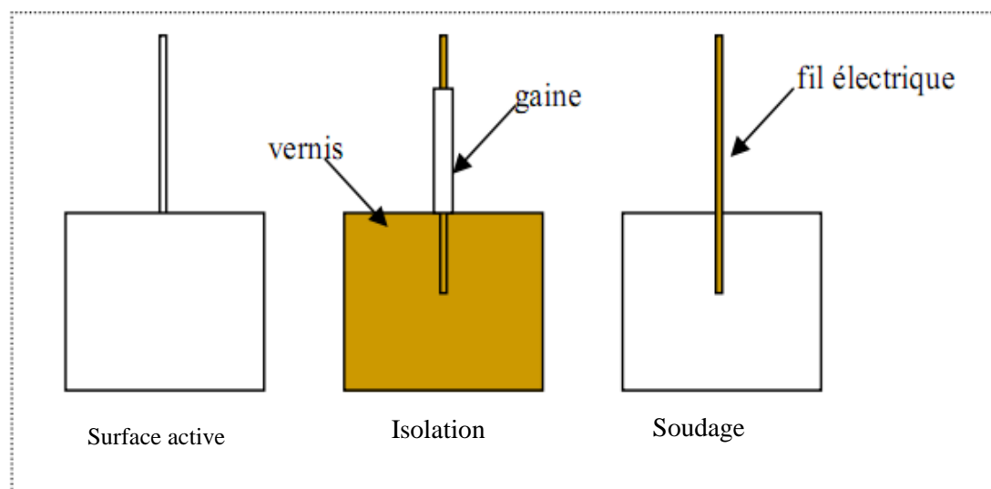
Figure III.2. Préparation des échantillons en acier DC04EK, pour les mesures potentiostatiques. . [45]
