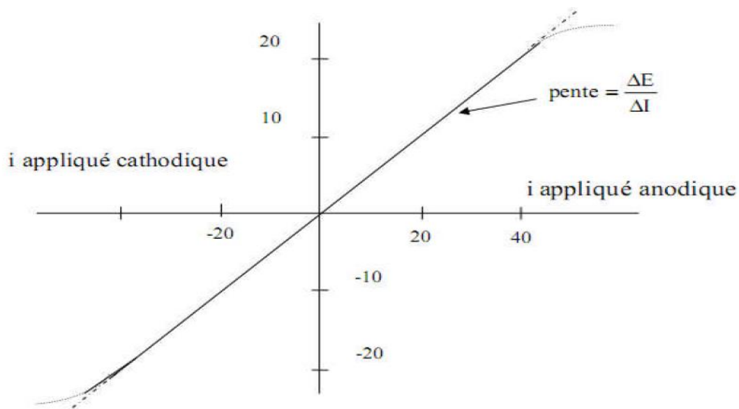
Figure I.8. Principe de la détermination graphique de la résistance de polarisation [52,53] .
