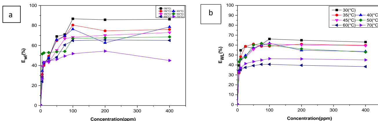
Figure IV.16. Efficacité d'inhibition en fonction de la concentration de l'acier DC06EK dans la solution H_2SO_4 (0,1 M), en présence de (a : Tryptophane+5ppm NaI, & b : Proline+5ppm NaI) à différentes températures.
