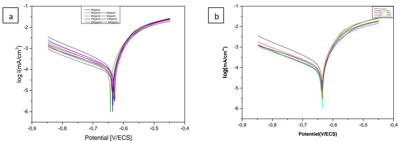
Figure IV.19. Courbes de polarisation de Tafel relatives à l'acier DC06EK dans H 2 SO 4 (0.1M) sans et avec addition de différentes concentrations de (a :Tryptophane + NaI & b :Proline + NaI ).
