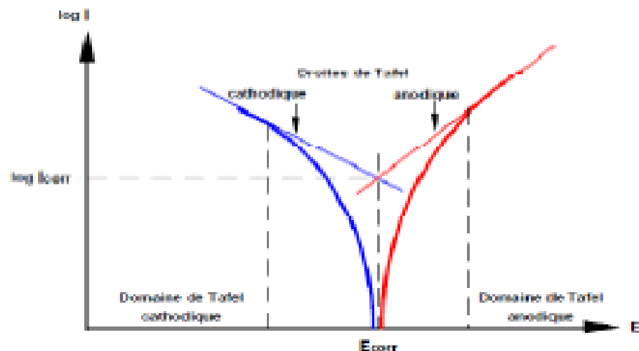
Figure I.7. Détermination des paramètres électrochimiques à partir des droites de Tafel pour un processus de corrosion sous contrôle d'activation pure. [51,52]
