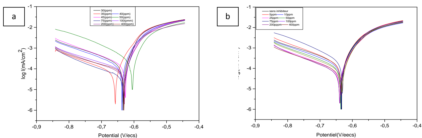
Figure IV.11. Courbes de polarisation de Tafel relatives à l'acier DC06EK dans H_2SO_4 (0.1 M) sans et avec addition de différentes concentrations en produits inhibiteurs (a :tryptophane, b :Proline) .
