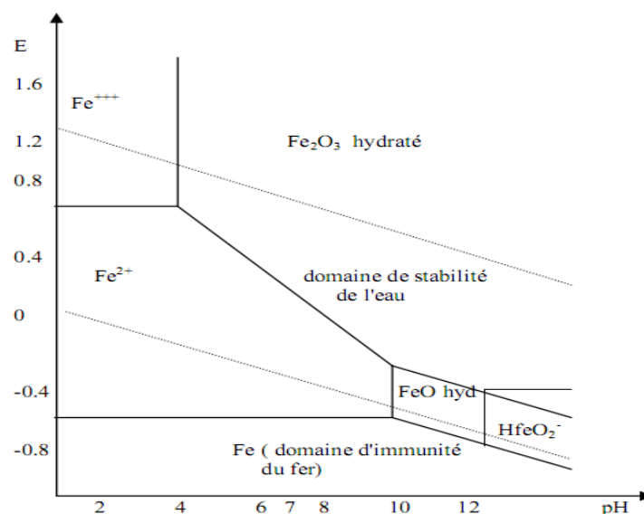
Figure I.2. Diagramme E- pH du fer dans l'eau pure à 25°C. [14]
