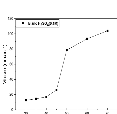
Figure IV.4. Vitesse de corrosion en fonction de la température de l'acier DC06EK dans la solution \text{H}_2\text{SO}_4 (0,1 M) sans inhibiteur.
