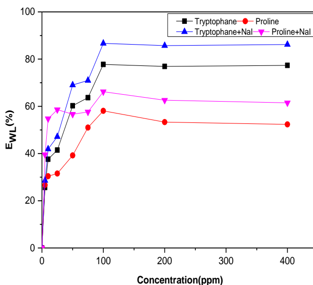
Figure IV.23. Efficacité d'inhibition de la corrosion de l'acier DC06EK dans H_2SO_4 (0,1 M) en fonction de la concentration des deux inhibiteurs ( Tryptophane et Proline ), en présence et en absence de 5 ppm en NaI
